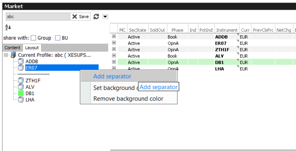
Fig. 42: Separators
