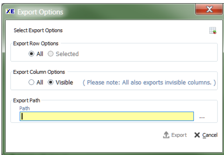
Fig. 31: Export Options
