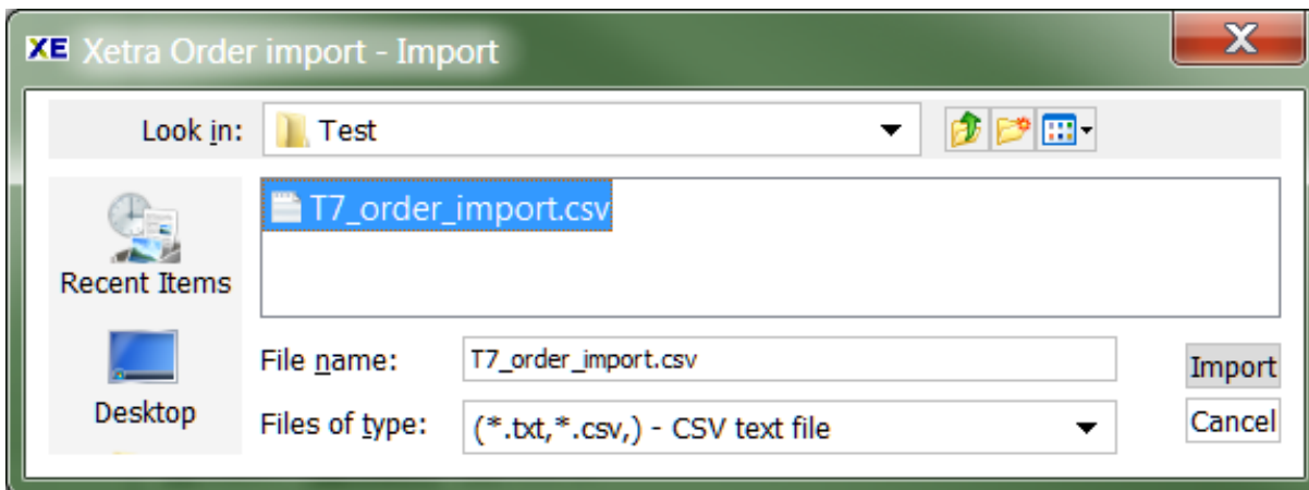
Fig. 30: Import Dialogue
